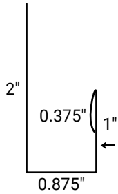
J-Channel • 30JC
