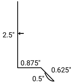
Drip Cap • 30DC
