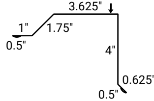
Denver Rake
