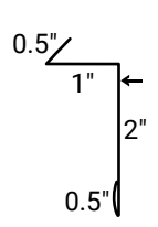
Reglet Flashing
