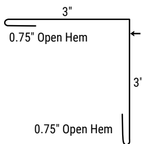
O/S Corner • 300C
